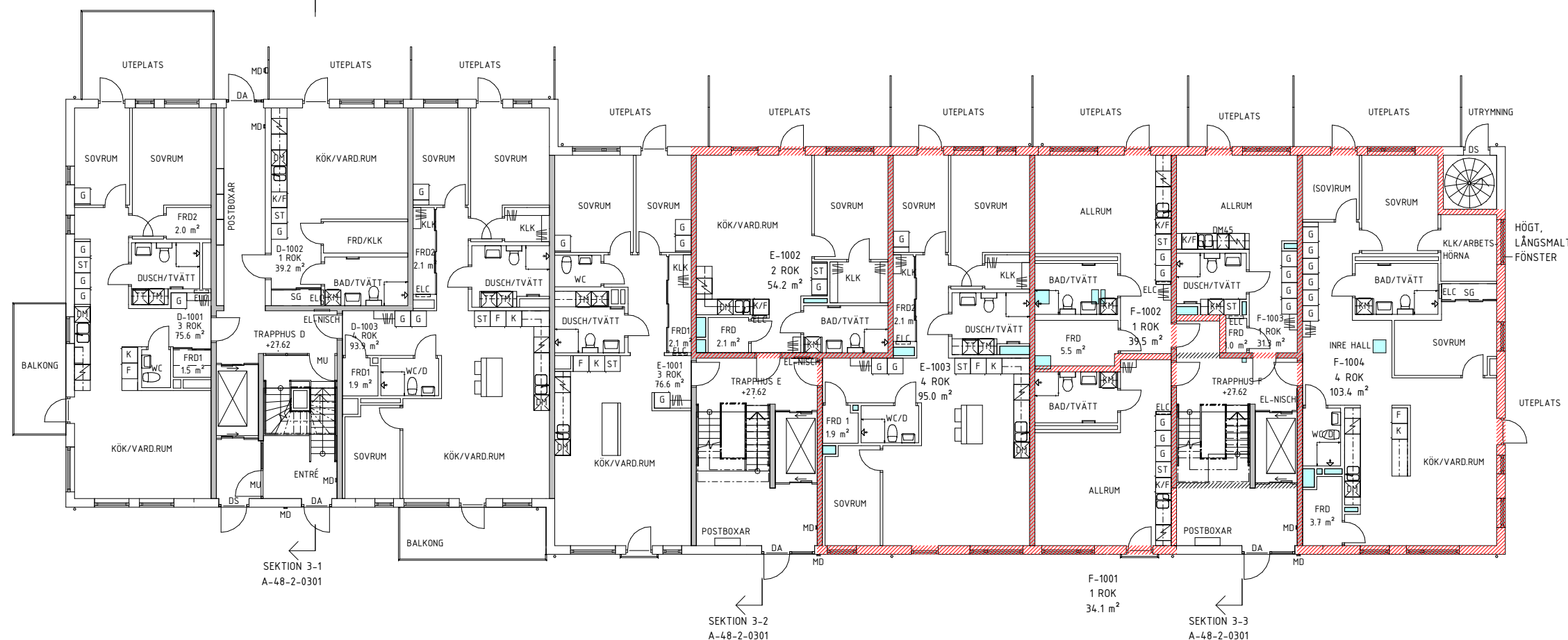
PLAN 10 (LSS-KONVERTERING)
