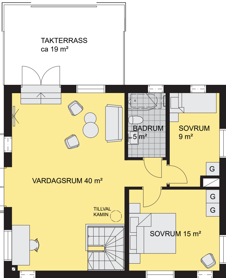
VÅNING 7
