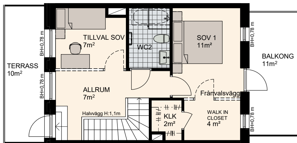
Våning 7, 42m 2
