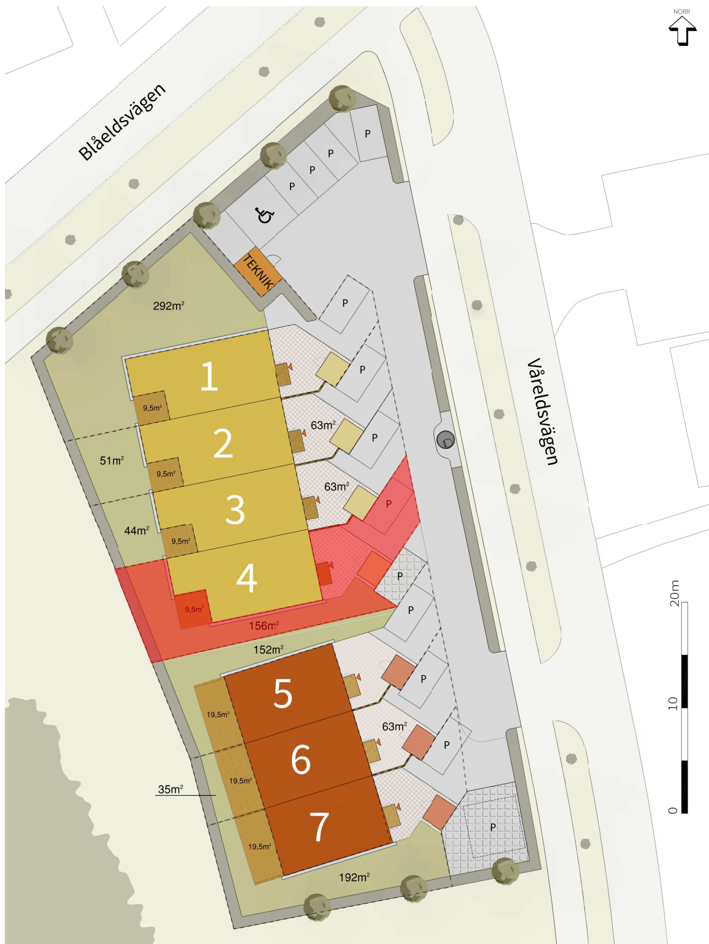
Situationsplan Brf Ängslunden, Sturefors Linköpings kommun 2020-04-07 Skala 1:250 (A3) Forum Arkitekter AB
