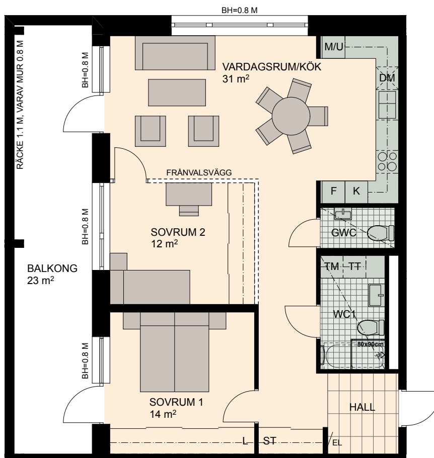
LÄGENHET MARKPLAN RUMSHÖJD 3.8 M
