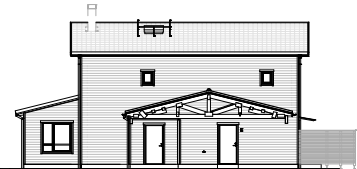
Fasad med förråd/carport
