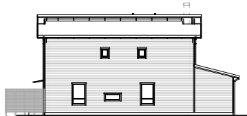
Fasad fri långsida (Hus 6)
