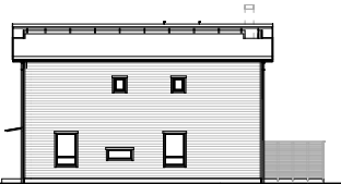
Fasad fri långsida (Hus 6)
