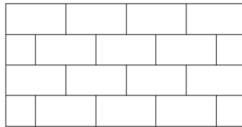
Halvstensförband
