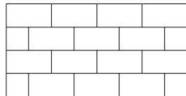
Halvstensförband
