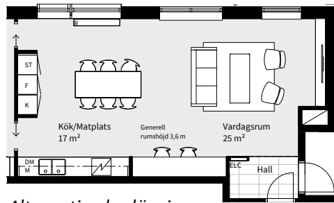
Alternativ planlösning
