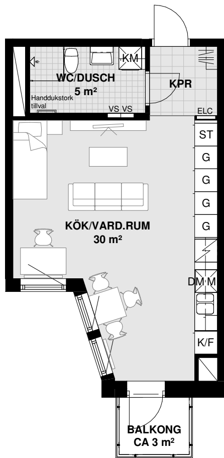
ALTERNATIV PLANLÖSNING
