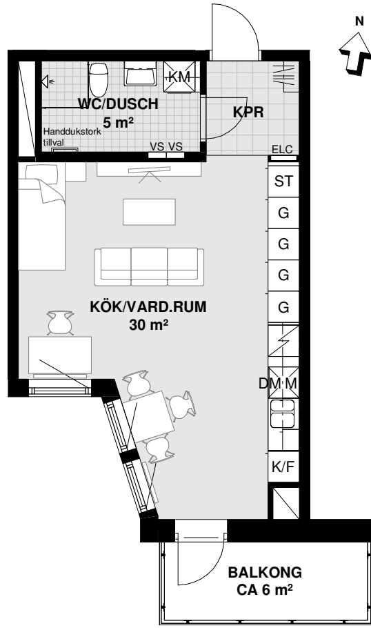
ALTERNATIV PLANLÖSNING
