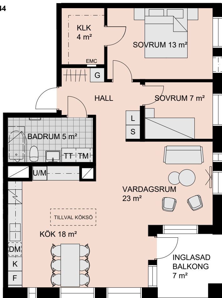
FÖNSTERSÄTTNING LGH. 8114 OCH 8134
