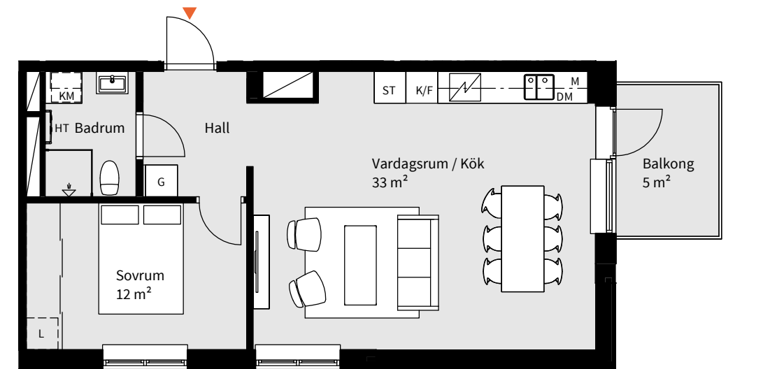
Lgh D1702 på våning 8 har en rumshöjd på 3,3 m.
