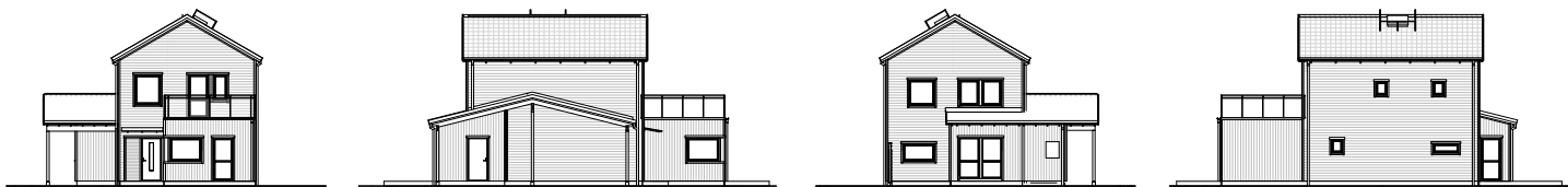
Fasad hus 2 - 4 + 6
